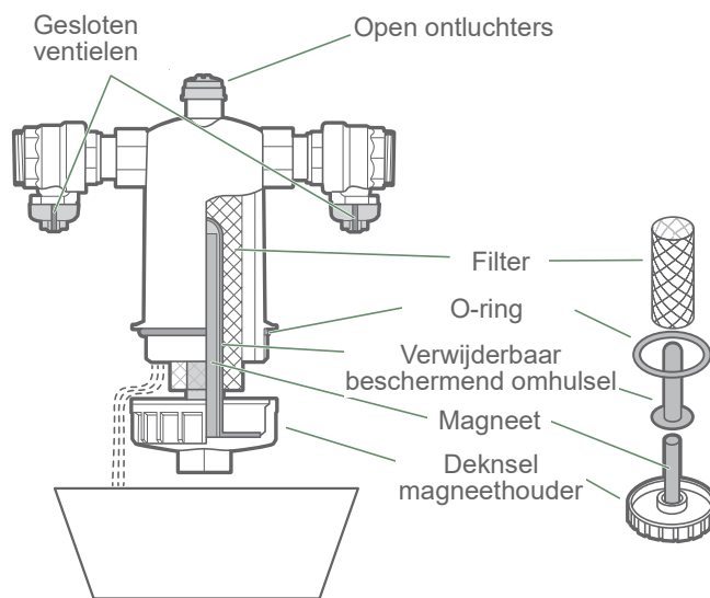
fig. 19 - Vuilfilter reinigen
