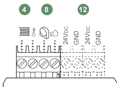
fig. 17 - Aansluitingen sensoren
