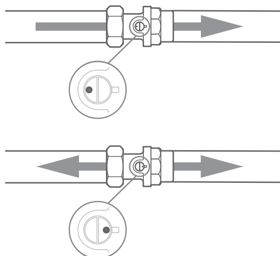
fig. 12 - Terugslagklep
