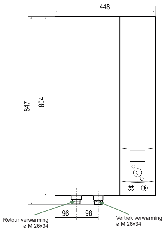
Vooraanzicht
