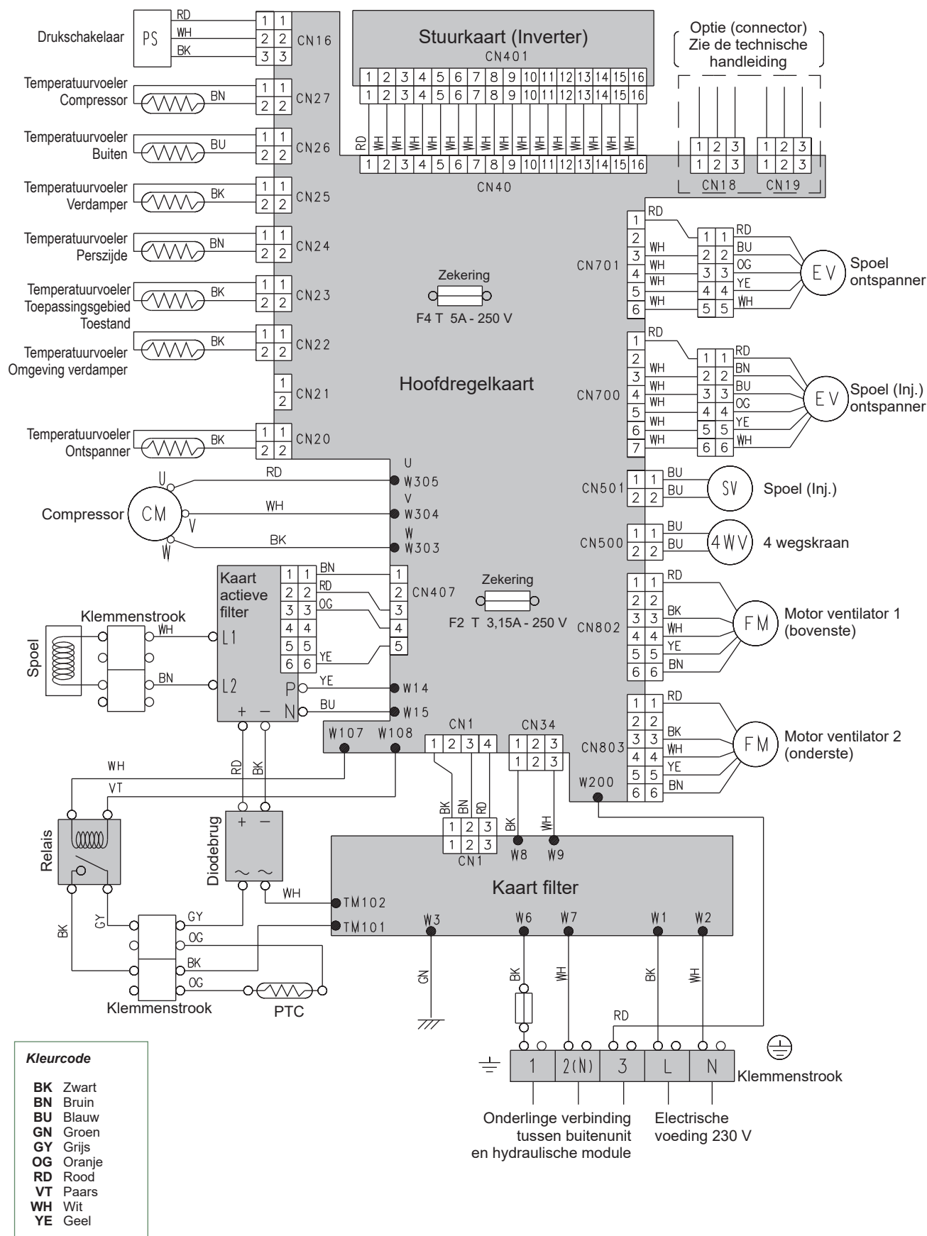
fig. 51 - Elektrisch kablering buitenunit model Alfa Excelsia A.I. éénfasig
