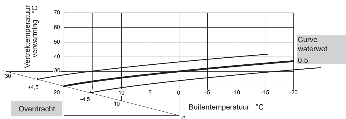
fig. 48 - Stookcurve voor de verwarming
