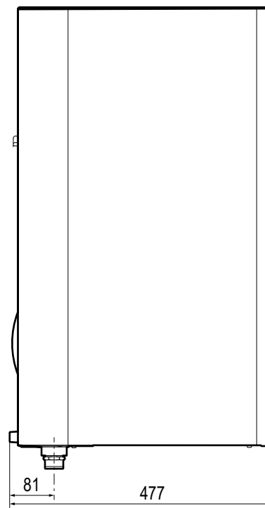
Zijaanzicht
