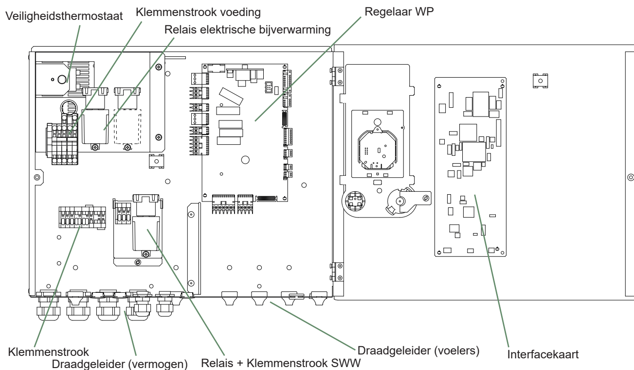
fig. 47 - Beschrijving van het elektriciteitskastje van de éénfasige hydraulische module
