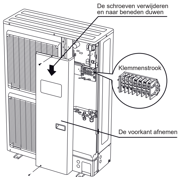
fig. 41 - Toegang tot de klemmenstrook van de driefasige buitenunit
