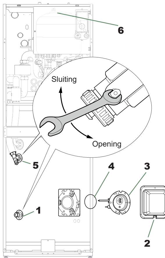
fig. 59 - De hydraulische module ledigen en/of Sanitaire boiler
