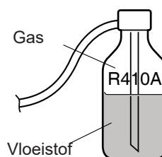
fig. 23 - Gasfles R410A
