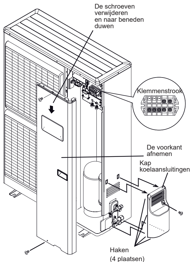
fig. 38 - Toegang tot de klemmenstrook van de buitenunit eenfasig
