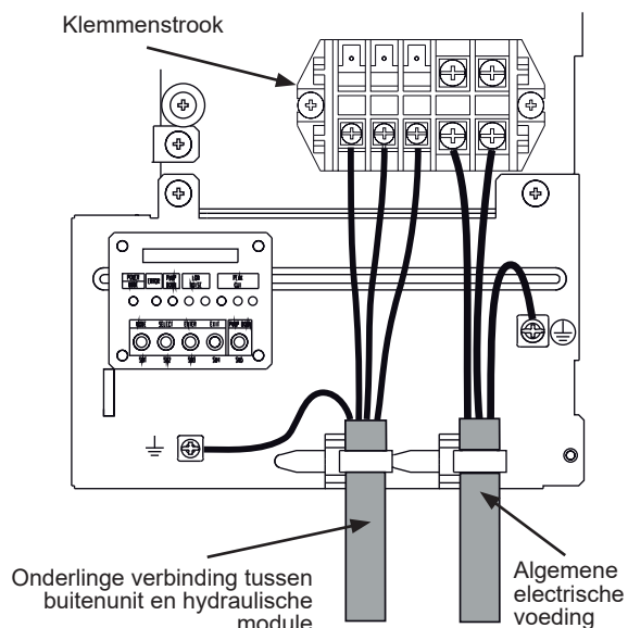
fig. 39 - Aansluitingen op de klemmenstrook van de éénfasige buitenunit
