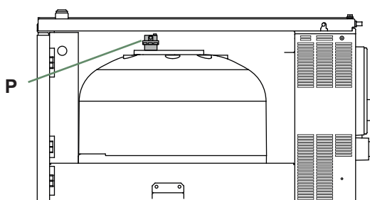
fig. 29 - Automatische ontluchter van de hydraulische module
