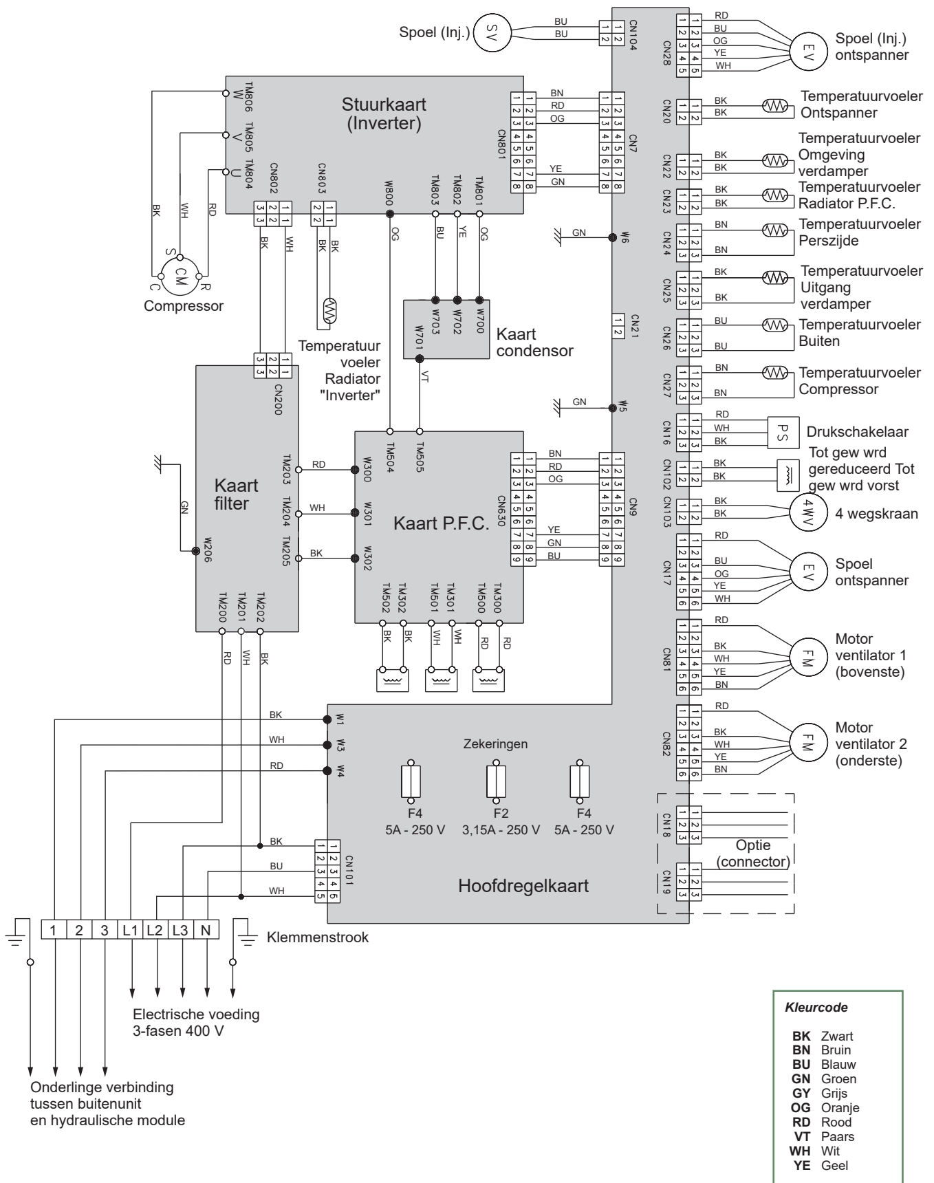
fig. 56 - Elektrische kablering buitenunit model Alfa Extensia Duo A.I. Driefasig
