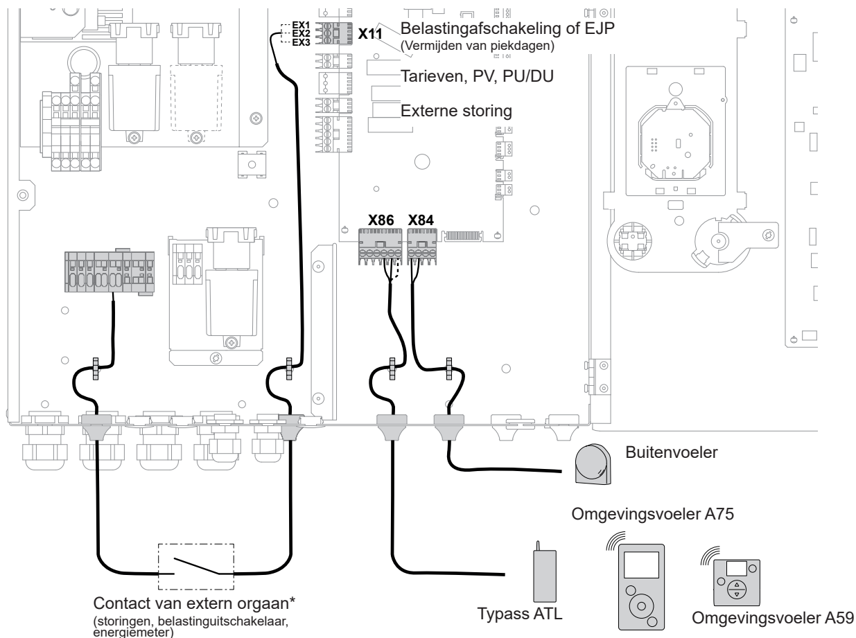
fig. 49 - Doorvoering van de kabels van de voelers
