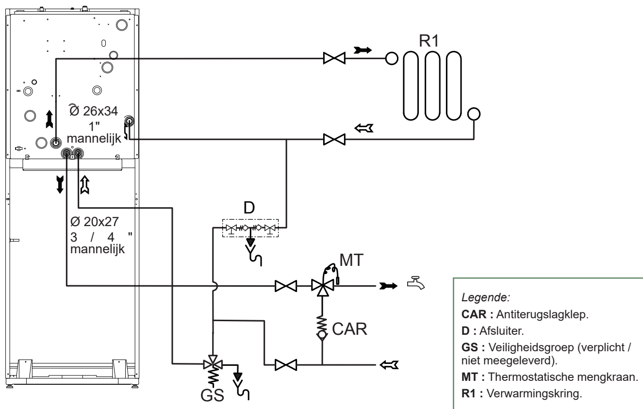
fig. 25 - Principeel hydraulisch schema
