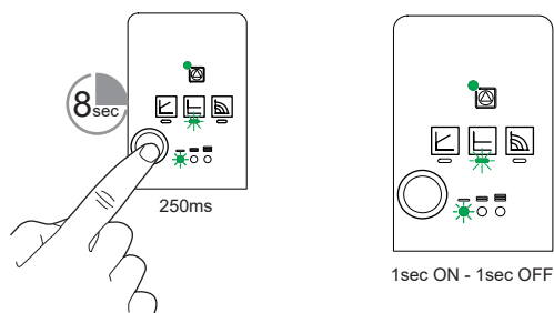
fig. 34 - Blokkering & ontgrendeling Circulatiepompinstellingen
