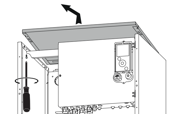
fig. 17 - Afnemen van het deksel
