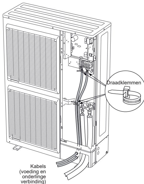
fig. 43 - Volttooiing van de verbinding van de driefasige buitenunit
