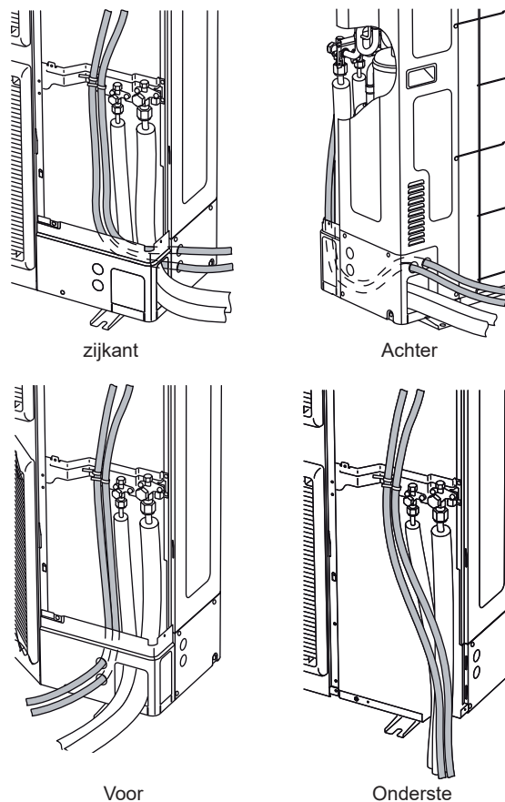
fig. 44 - Doorgang van de kabels en koeltechnische verbindingen van de driefasige buitenunit
