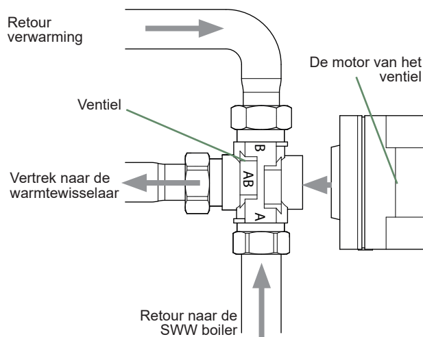
fig. 60 - Montage van de richtingskraan
