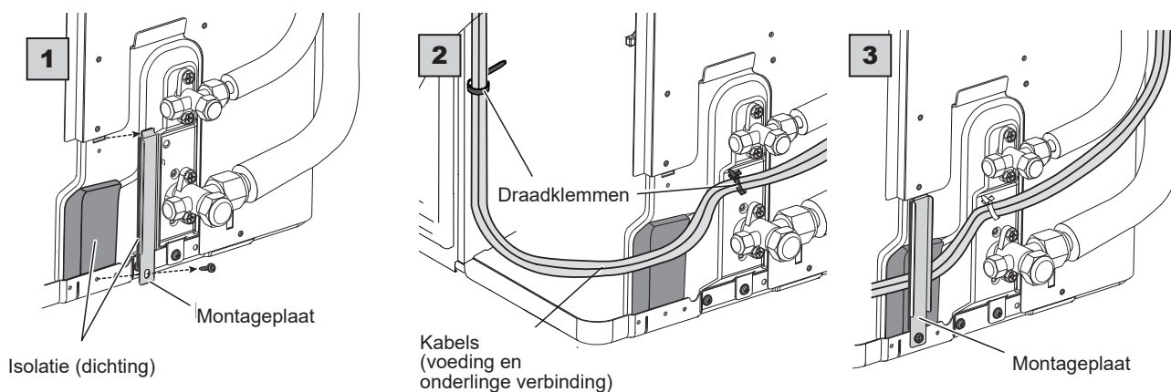
fig. 38 - Toegang tot de klemmenstrook van de buitenunit eenfasig
