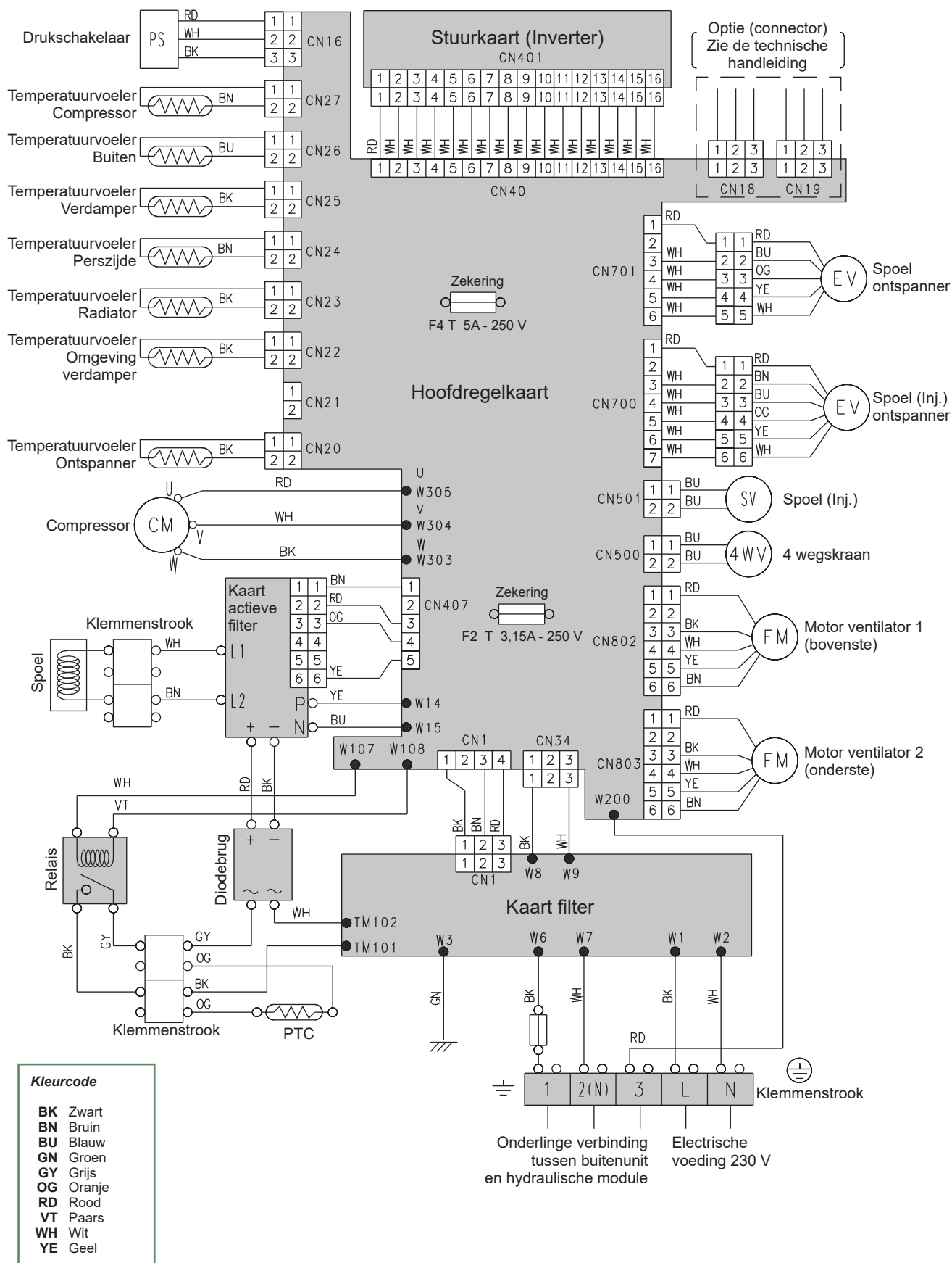
fig. 55 - Elektrische kablering buitenunit model Alfa Excelsia Duo A.I. éénfasig
