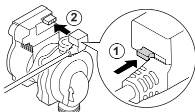
fig. 31 - Aansluiting van de circulatiepomp
