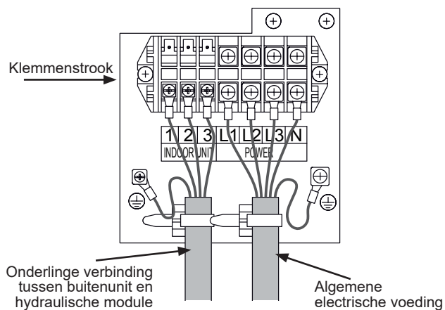
fig. 42 - Aansluitingen op de klemmenstrook van de buitenunit driefasig
