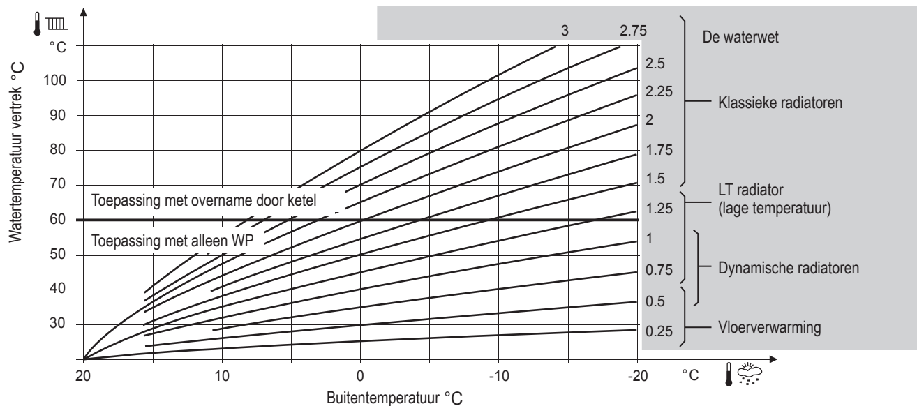
fig. 52 - Stookcurve voor de verwarming (lijn 720)
