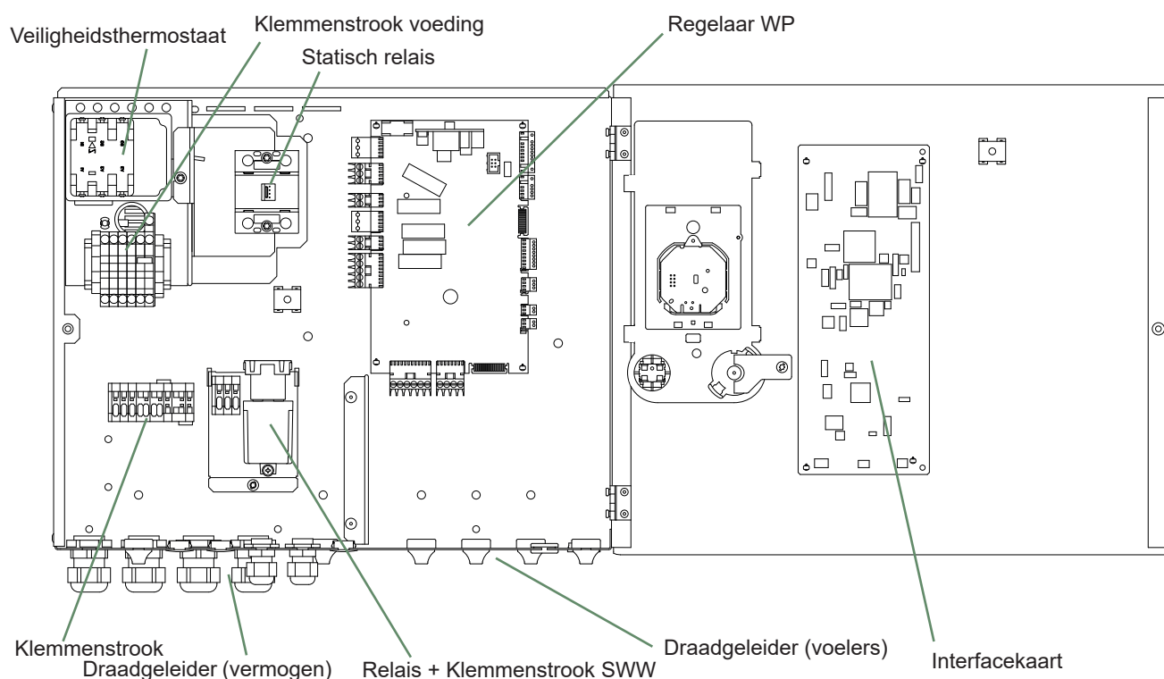
fig. 46 - Beschrijving van het elektriciteitskastje van de driefasige hydraulische module
