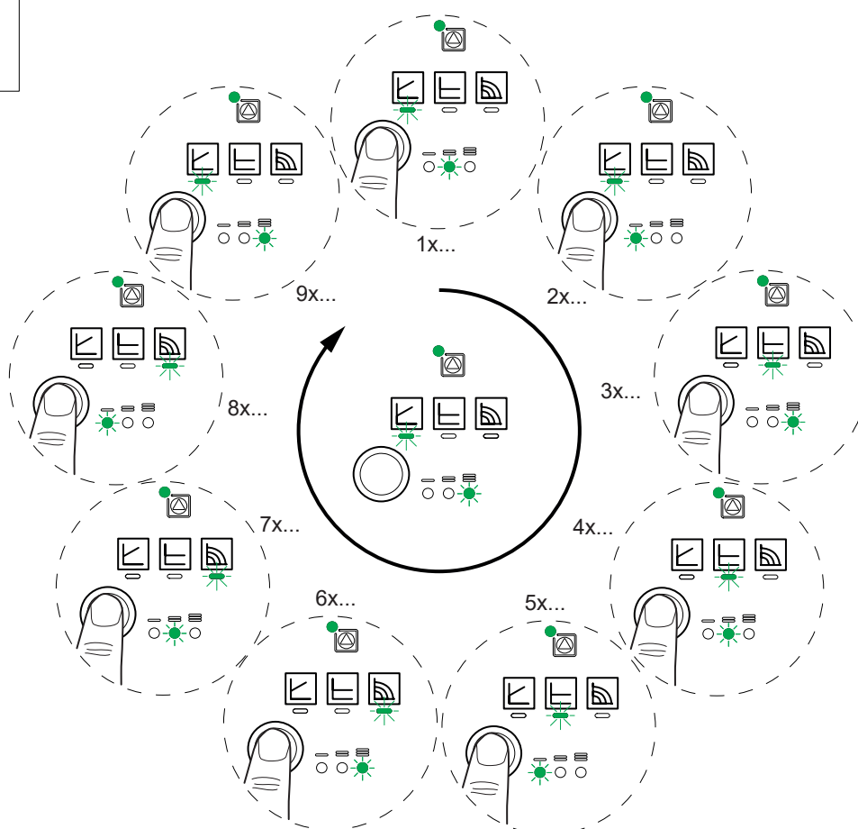
fig. 35 - Circulatiepomp instellingen
