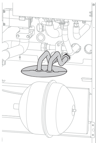
fig. 26 - Montage van de SWW-leidingen
