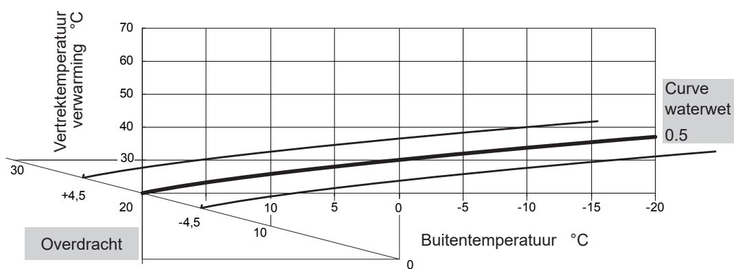
fig. 53 - Overdracht van de stookcurve voor de verwarming (lijn 721)
