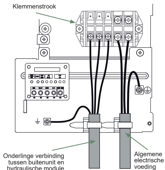
fig. 35 - Aansluitingen op de klemmenstrook van de éénfasige buitenunit
