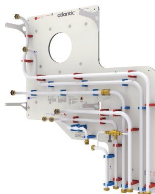
Prefab leidingwerk kit Simplifix
